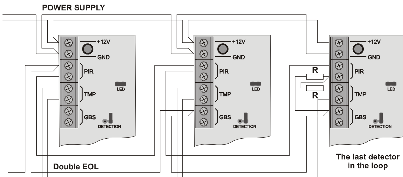
Kelių JS-20 "Largo" jutiklių jungimo pavyzdžiai su dviguba galinių varžų grandine (Pagalbiniai GBS kontaktai yra laisvi, praverčiantys laidų prijungimui)
